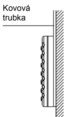
Obr. 12: Povrchová instalace kabelu
