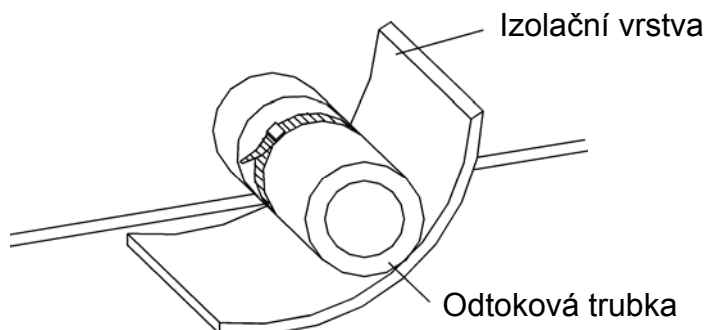
Obr. 9: Tepelná izolace odtokové trubky.
