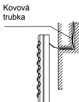
Obr. 13: Skrytá instalace kabelu
