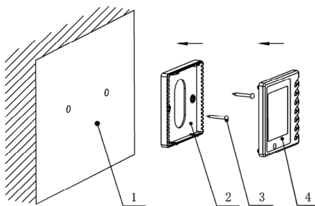
Obr. 14: Postup při instalaci
